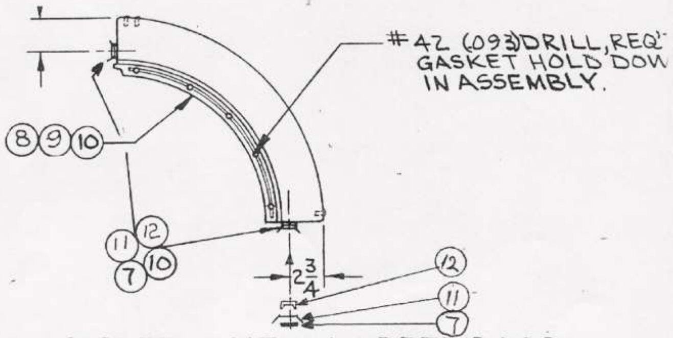
GASKET LOCATION-UPPER DOOR
